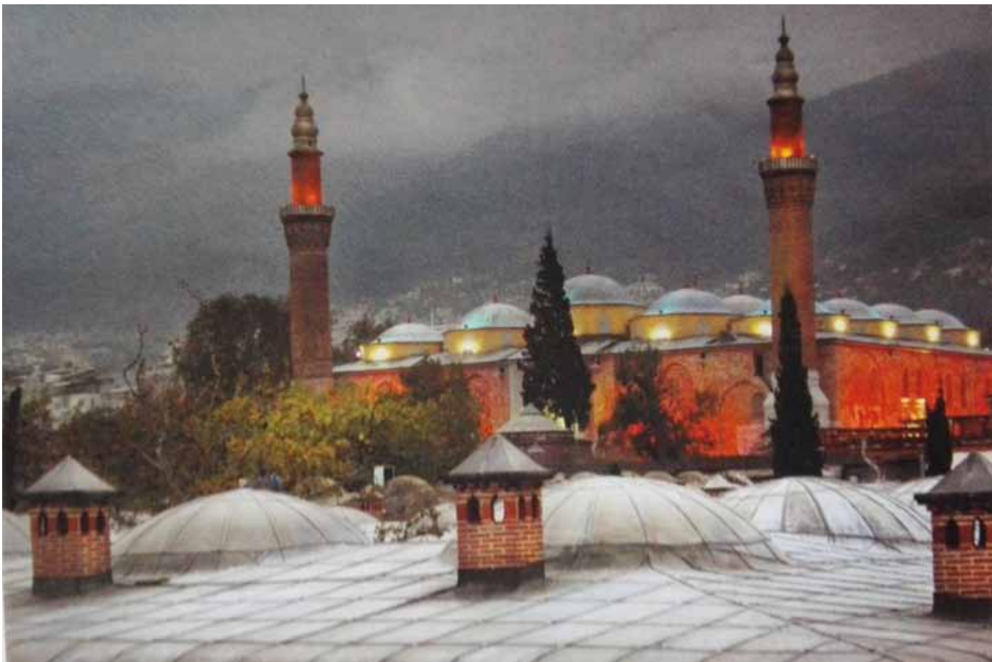
20-kupolinen ULU-moskeija.
